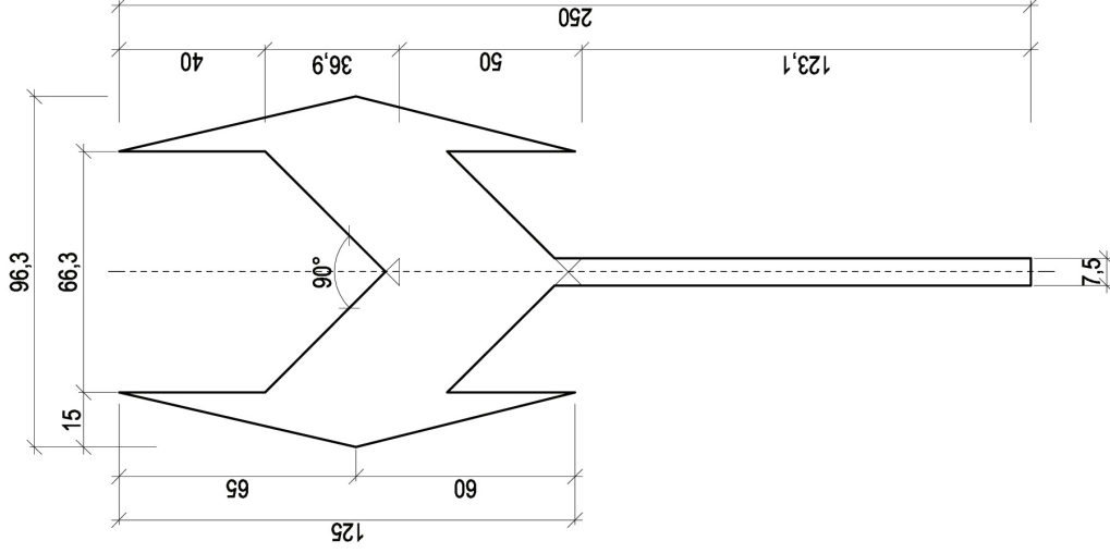
P-8g mini strzałka kierunkowa w lewo lub w prawo
