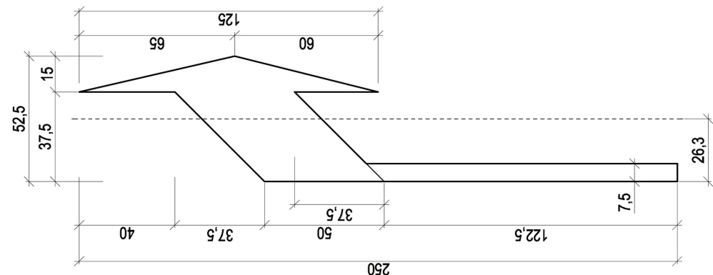
P-8d mini strzałka kierunkowa w prawo
