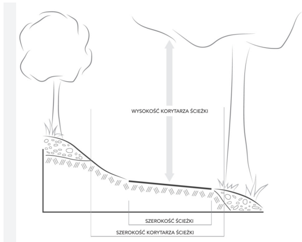
SCHEMAT 49. Przestrzeń zajmowana przez zrównoważoną trasę rowerową.
