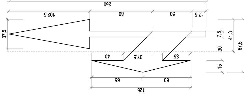
P-8e mini strzałka kierunkowa na wprost lub w lewo
