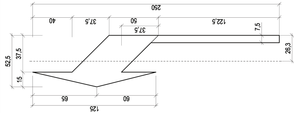
P-8b mini strzałka kierunkowa w lewo
